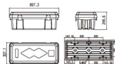
灭火器箱 型号: NG15050 灭火器4-8kg 材料: 塑料 重量: 3.7kg Type Number: NG15048 Material: PP Weight: 3.7kg
