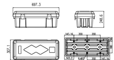
灭火器箱 型号: NG15050 灭火器4-8kg 材料: 塑料 重量:3.7kg Type Number:NG15048 Material:PP Weight:3.7kg
