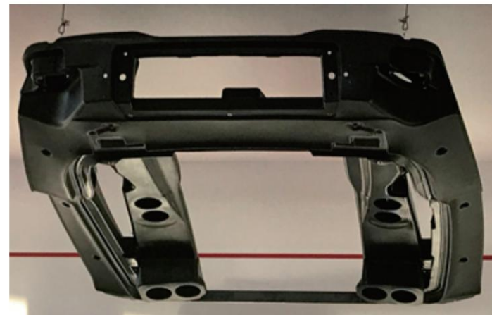
带空调通风管的拖拉机顶棚
